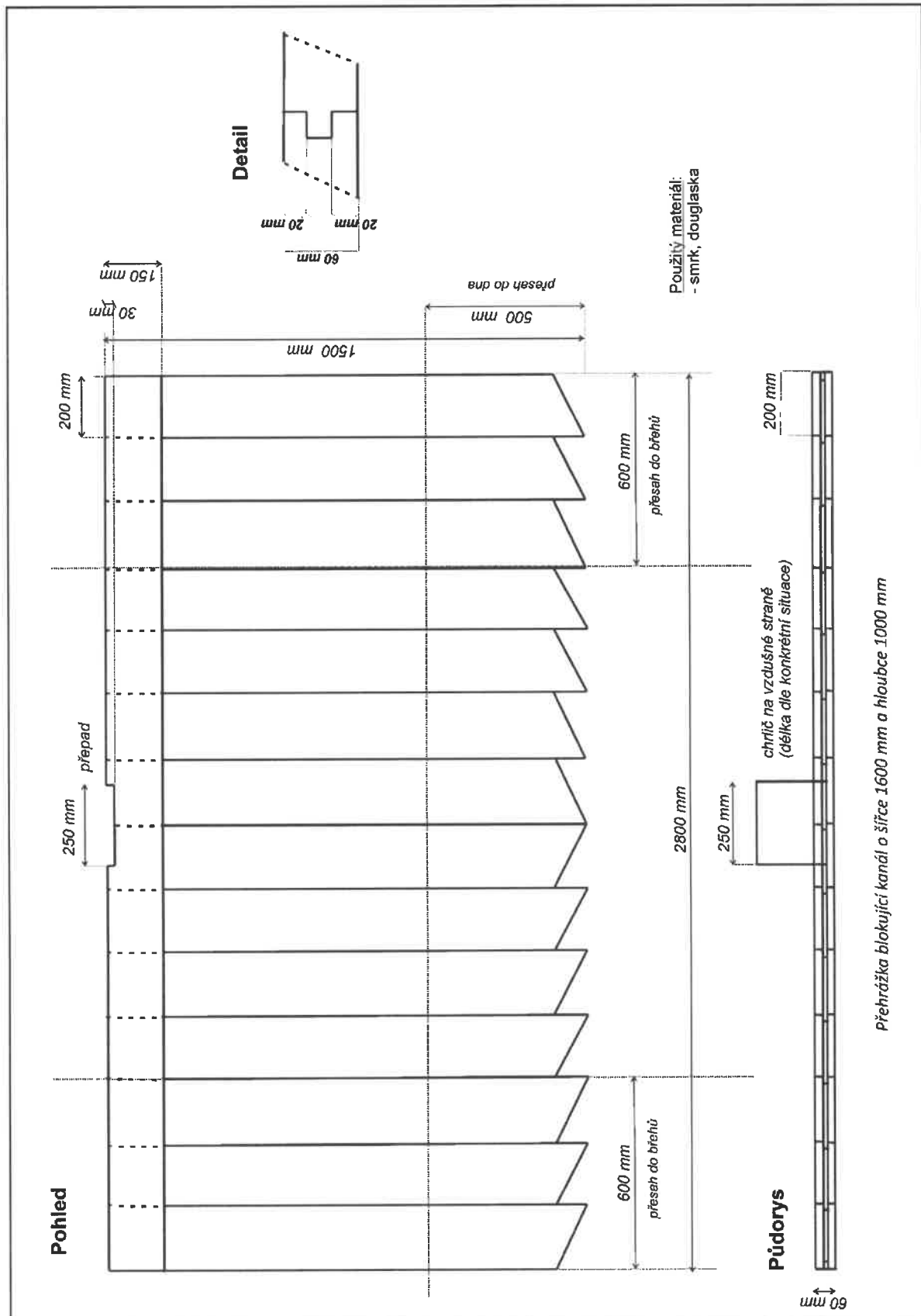
Obr. 6a: Schéma vertikálně instalované přehrážky z opracovaných fošen, spojení „pero-drážka“.
