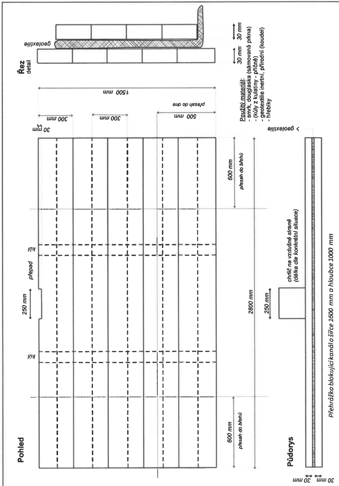
Obr. 2: Schéma zdvojené přehrážky z vodorovně instalovaných prken.
