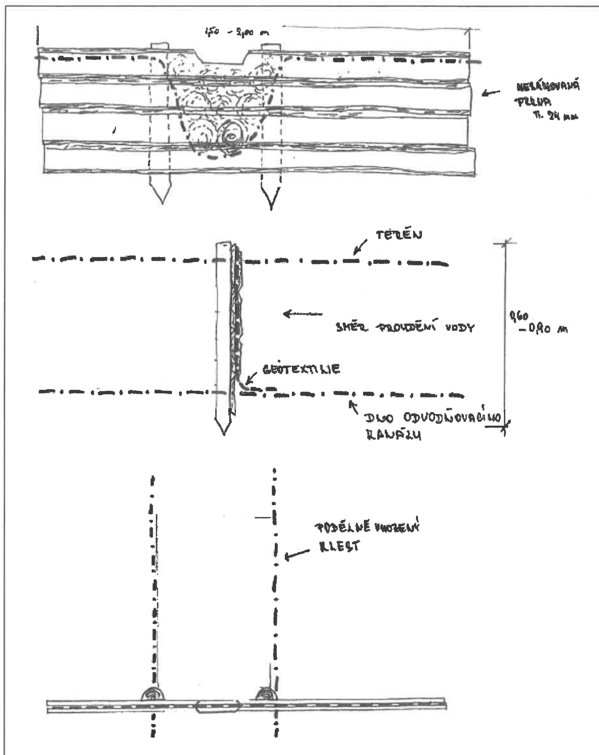
Obr. 5: Jednoduchá přehrážka ze smrkových prken
