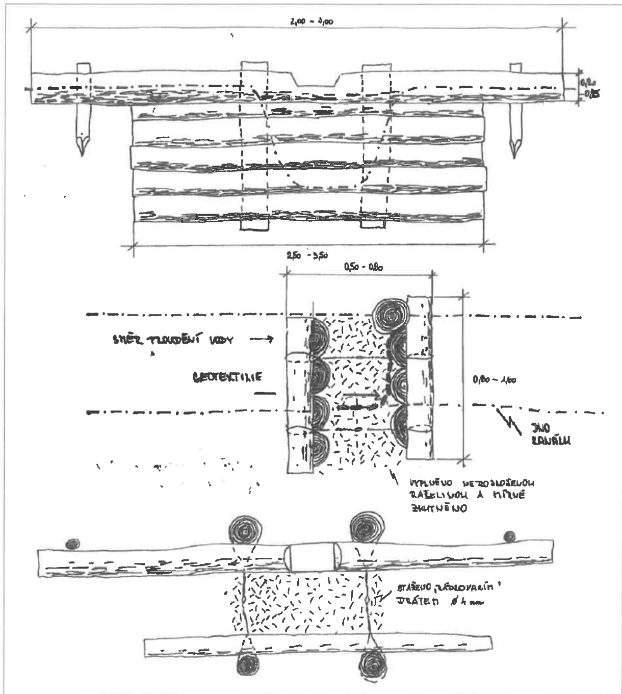
Obr. 3: Dvojitá přehrážka srubového typu ze smrkové kulatiny. Rašelina v meziprostoru je zhutněna lopatou nebo stlačena lžící bagru. Zdroj: RNDr. Vladimír Zýval st.
