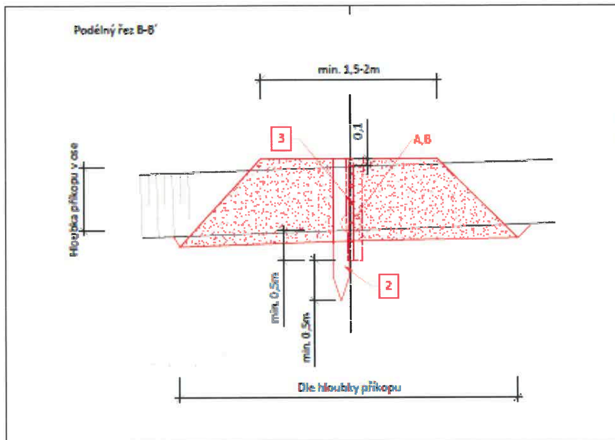
Obr. 7: Schematické znázornění obsypu přehrážek zeminou. Zdroj: RNDr. Ivana Bufková, Ph.D.
